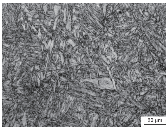
图 B.4 回火马氏体组织,放大倍数 500 \times
