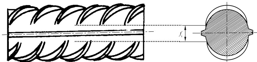
标引符号说明: f 1 ——横肋末端间隙。
